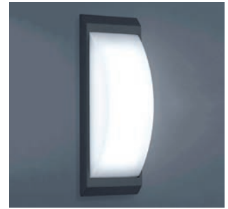
LED-Fassadenleuchte Aluminium/Kunststoff, graphit/opal B 100, H 20, T 40 inkl. 8 W/510 lm/3000 K UV- und witterungsbeständig
